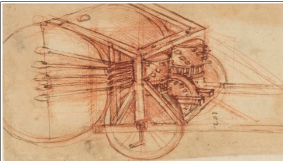
Tamburo Militare Meccanizzato - Codice Atlantico foglio n° 837
